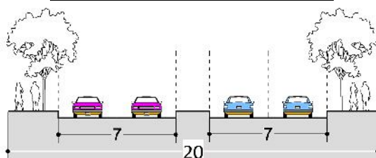
Perfil Máximo Acceso Rucalhue
