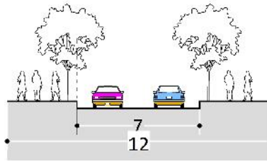
Perfil Máximo Puerto Saavedra
