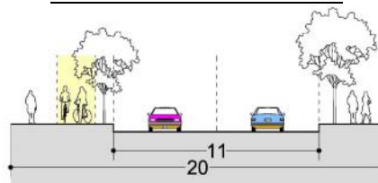
Perfil Máximo Marco Polo
