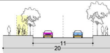
Perfil Máximo Acceso Ifarle Poniente
