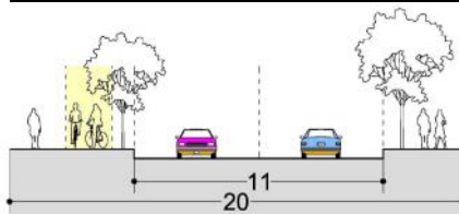
Perfil Máximo Probable Borderío
