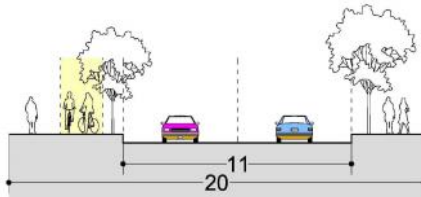
Perfil Máximo Gran Bretaña
