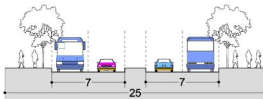
Perfil Máximo Probable Avenida Arteaga Alemparte
