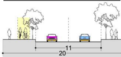
Perfil Máximo Padre Las Casas.
