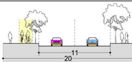
Perfil Máximo Probable Avenida Hualpén
