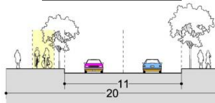
Perfil Máximo Cañete
