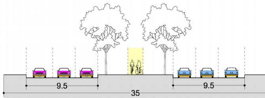
Perfil Máximo Probable Camino a la Desembocadura
